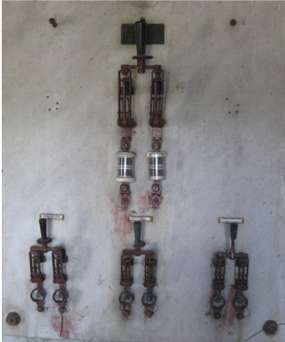
Quadro generale
