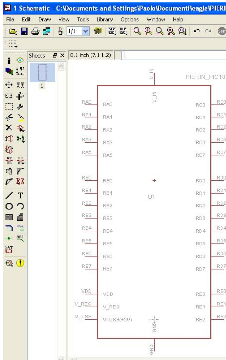
Pierin PIC18 - Simbolo per schematico con EAGLE
