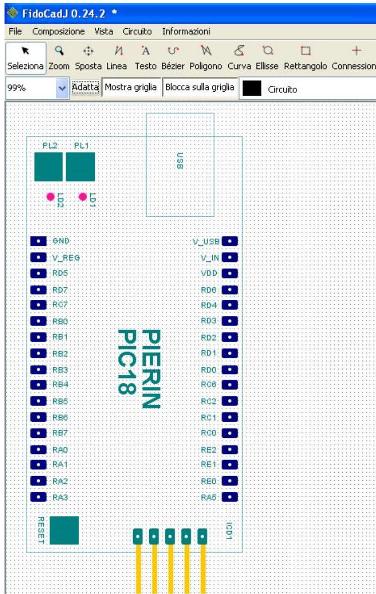
Pierin PIC18 - Impronta per PCB con FidoCADJ
