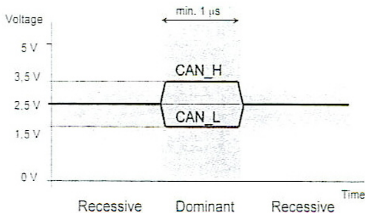
Figura 2 tensione sulle linee H ed L
